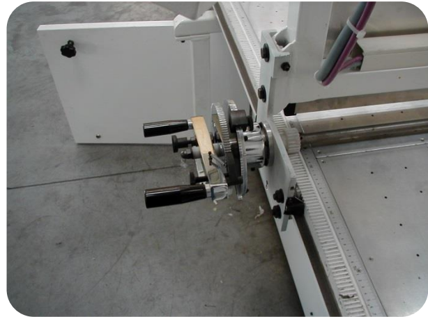
Sistema meccanico ripetitivo Mechanical repeating system
